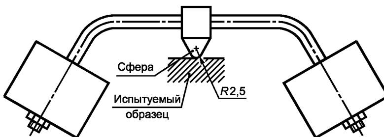
Рисунок 1 — Установка для испытания на теплостойкость
