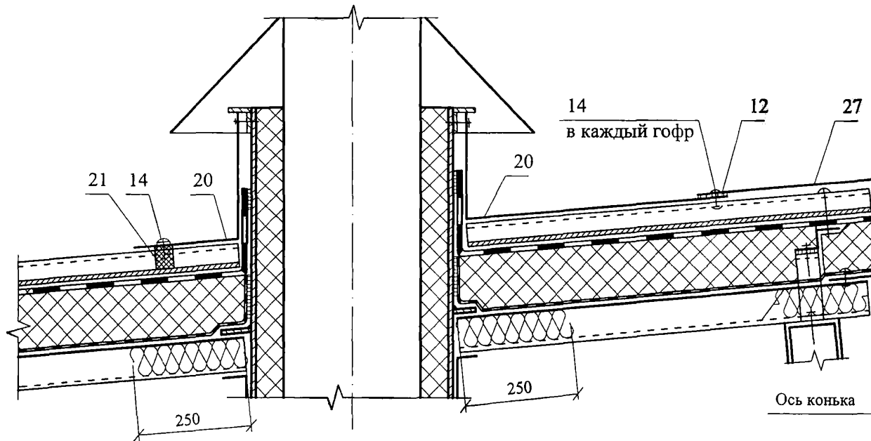
1 - 1 (узел 5)
