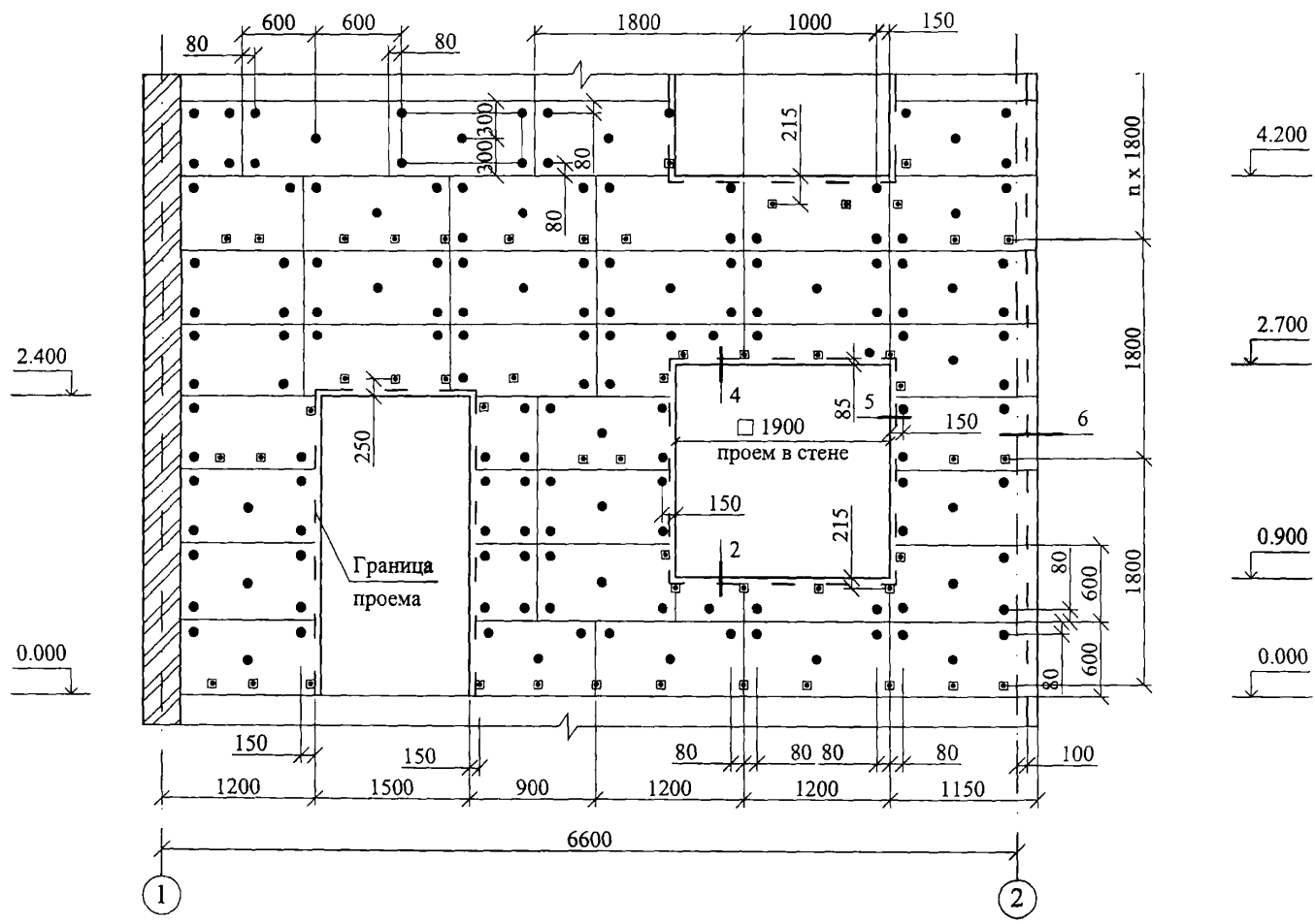
СХЕМА раскладки плит теплоизоляции
