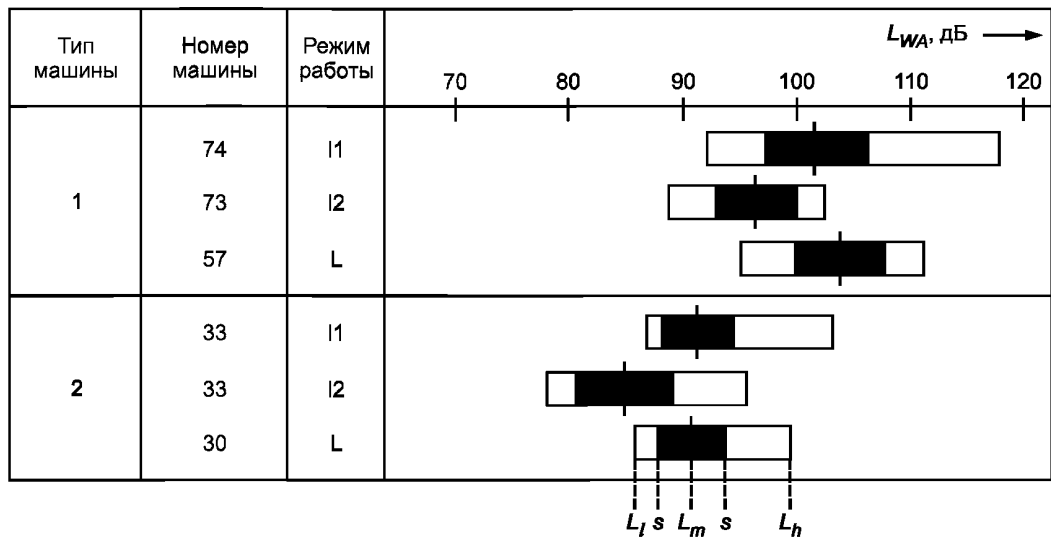
I1 — режим холостого хода при максимальной скорости; I2 — режим холостого хода при номинальной скорости; L — нагрузка при заданном режиме работы с рабочим инструментом; s — стандартное отклонение; L_l — наименьший уровень; L_m — средний уровень; L_h — наибольший уровень
