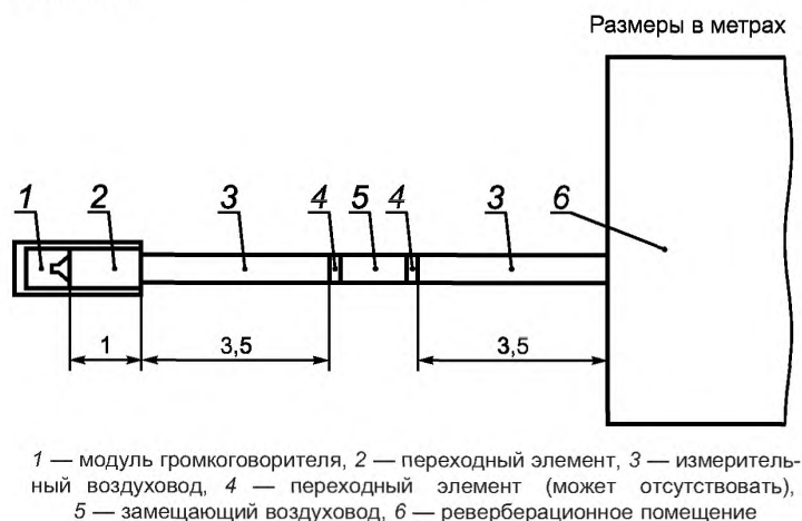
Рисунок 1 — Испытательная установка
