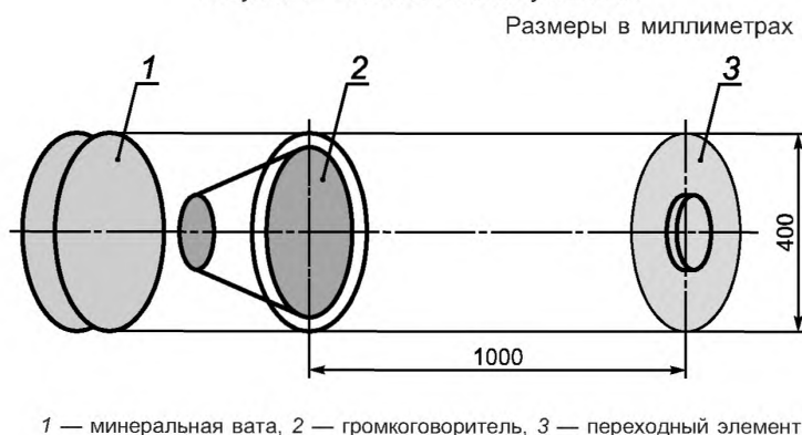
Рисунок 2 — Источник звука
