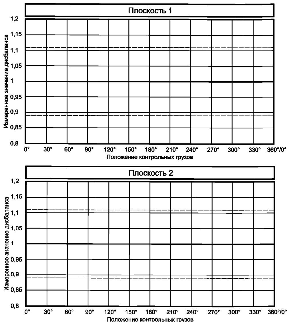
Рисунок 11 — График для оценки минимально достижимого остаточного дисбаланса
