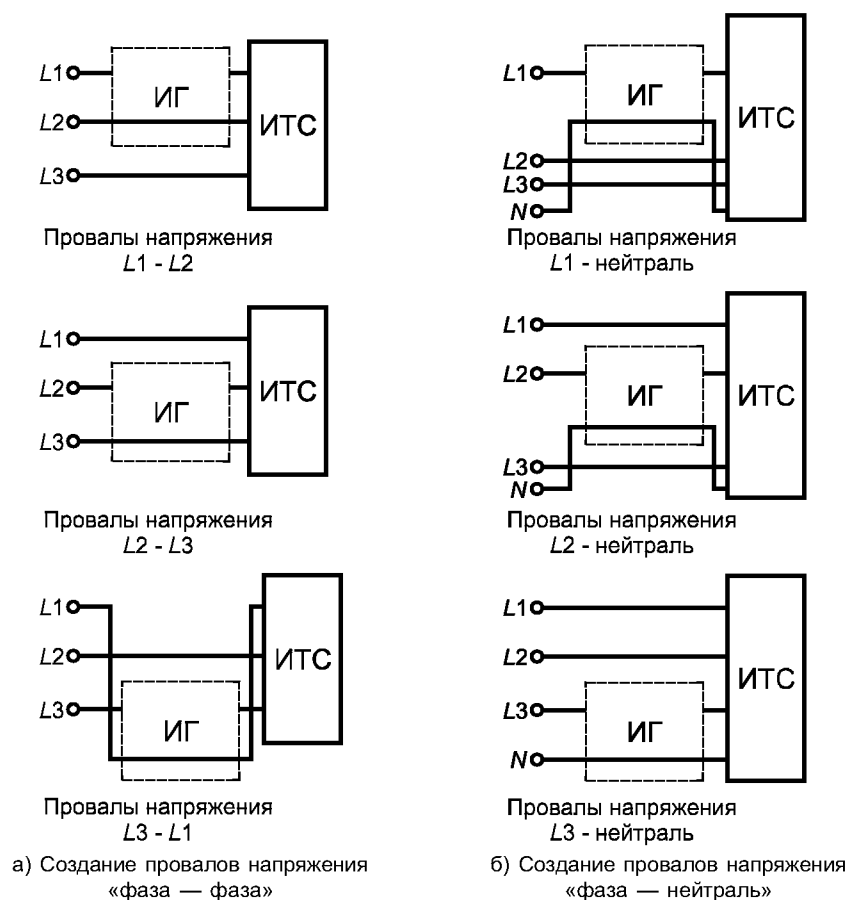
Рисунок Г.2 — Применение ИГ, приведенного на рисунке Г.1, для создания векторов напряжения электропитания при испытаниях трехфазных систем (допустимый метод 1) (см. рисунки 3б), в), В.1, В.2)
