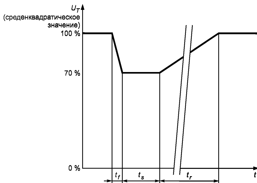
Рисунок 1 — Провал напряжения 70 % U_T
