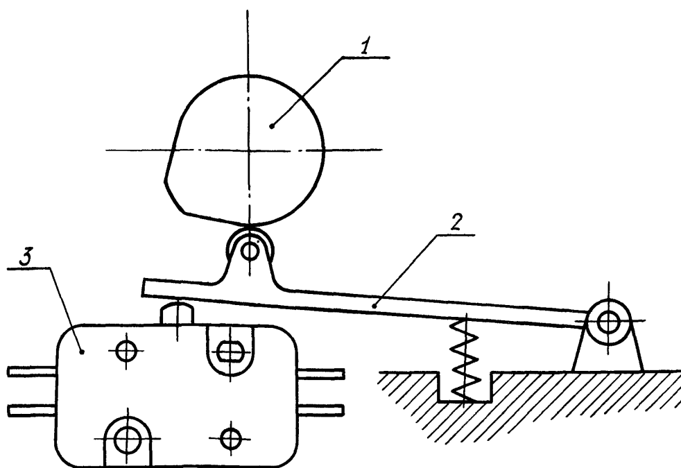
1 - кулачок; 2 - элемент промежуточный; 3 - микровыключатель
