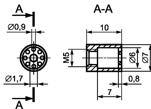
а) газовая горелка
