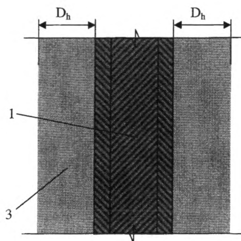
Рис. 4 а. Схема укладки и параметры теплоизоляции ПЕНОПЛЭКС® при устройстве ленточной опоры 1 — ленточная опора; 2 — фундамент; 3 — теплоизоляционный слой ПЕНОПЛЭКС®; 4 — песчано-гравийная смесь; 5 — отмостка; 6 — песчаная подготовка под отмостку
