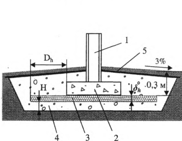
Рис. 4. Схема укладки и параметры теплоизоляции ПЕНОПЛЭКС® в фундаментах отдельно стоящих опор 1 — опора; 2 — фундамент; 3 — теплоизоляционный слой ПЕНОПЛЭКС®; 4 — песчано-гравийная смесь; 5 — водоупорный слой
