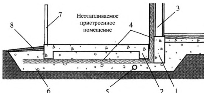
Рис. 5. Соприжение отапливаемого здания с холодной пристройкой
