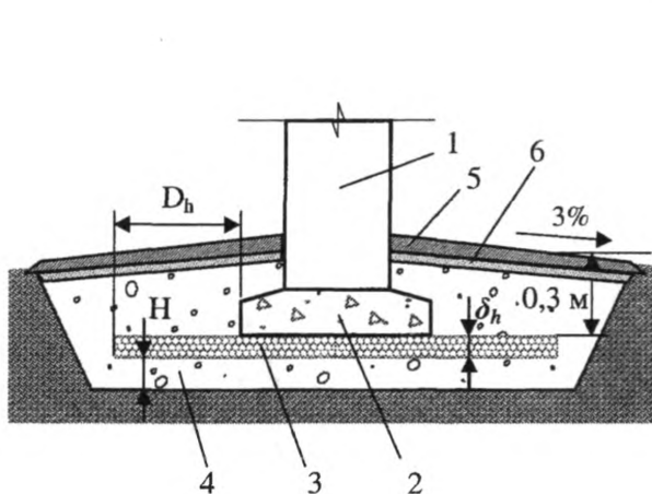
Рис. 4. Схема укладки и параметры теплоизоляции ПЕНОПЛЭКС® в фундаментах отдельно стоящих опор 1 — опора; 2 — фундамент; 3 — теплоизоляционный слой ПЕНОПЛЭКС®; 4 — песчано-гравийная смесь; 5 — водоупорный слой
