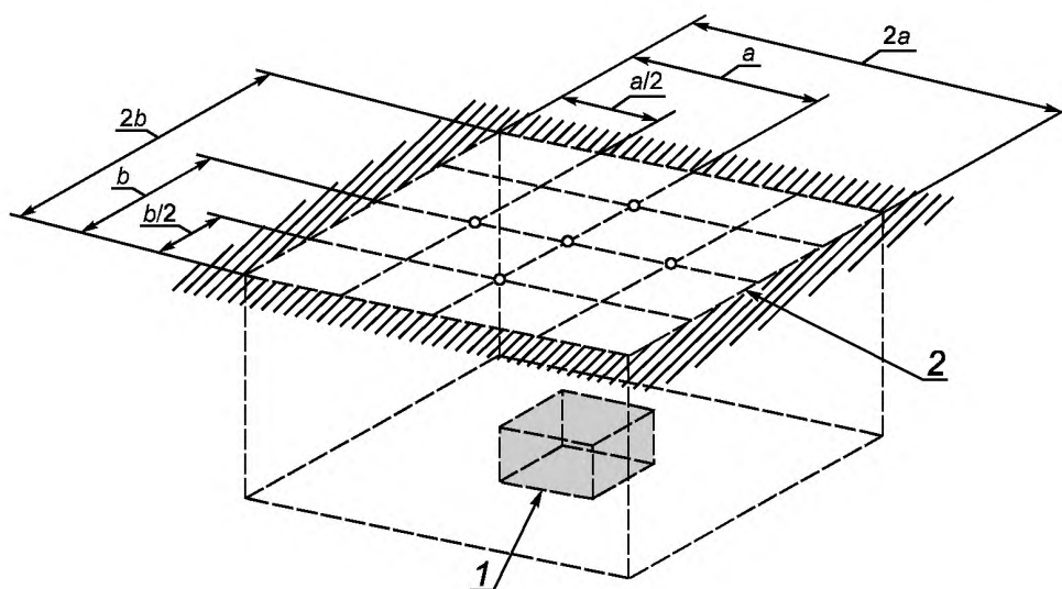
1 — огибающий параллелепипед; 2 — измерительная поверхность
