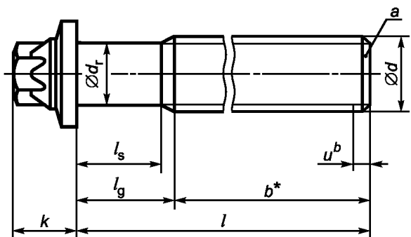
б) Болты длиной < 10d
