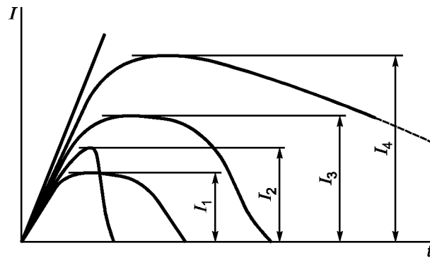
Рисунок 15 — Определение ожидаемого тока отключения после проведения первой калибровки при токе, меньшем номинальной отключающей способности (см. 8.3.4.1.8, перечисление b)
