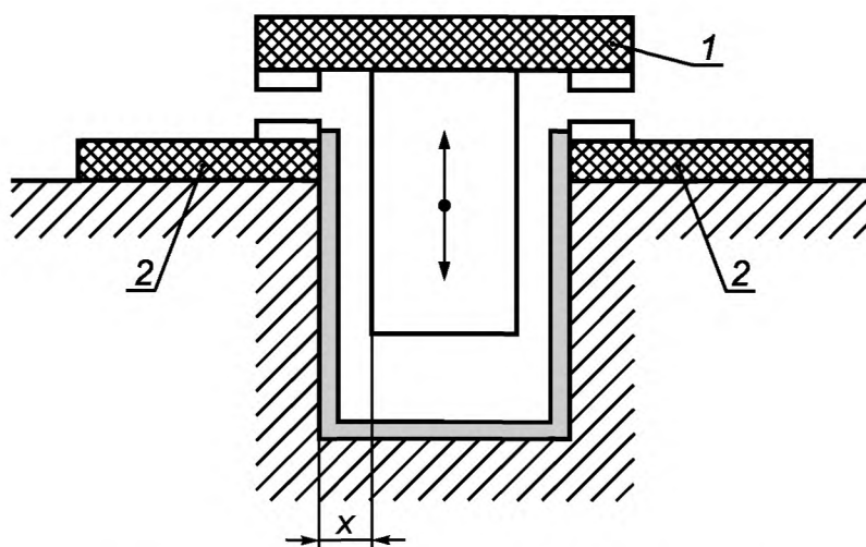
1 — подвижный контактный мостик; 2 — неподвижные контакты
