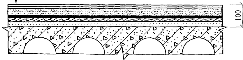
Рисунок 1 – Пол из линолеума на теплозвукоизолирующей подоснове
