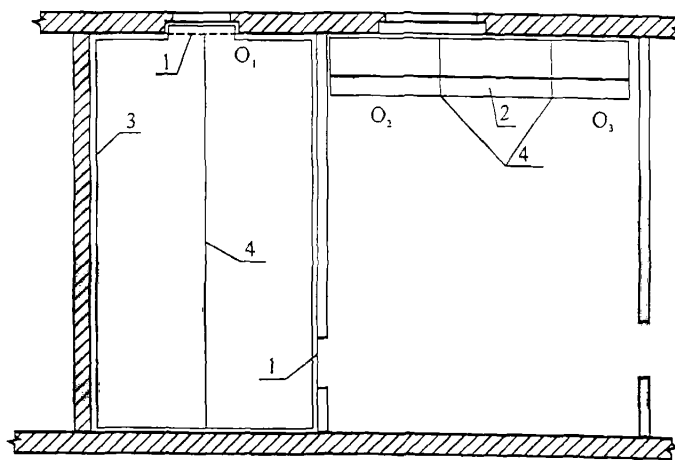
2.22 Схема организации рабочего места при устройстве полов из сваренного в ковры линолеума ПВХ на теплозвукоизолирующей подоснове приведена на рисунке 14.
