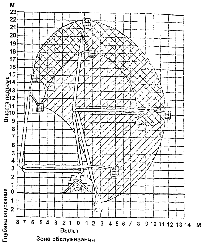
рис. 16. Автогидроподъемник АГП-22.04.
