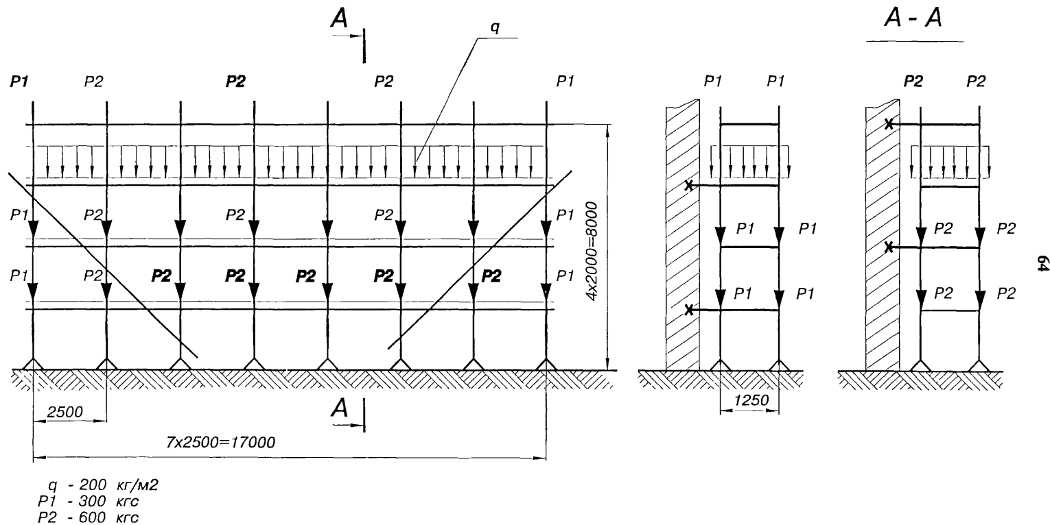
рис. 32. Схема допускаемых нагрузок на леса.
