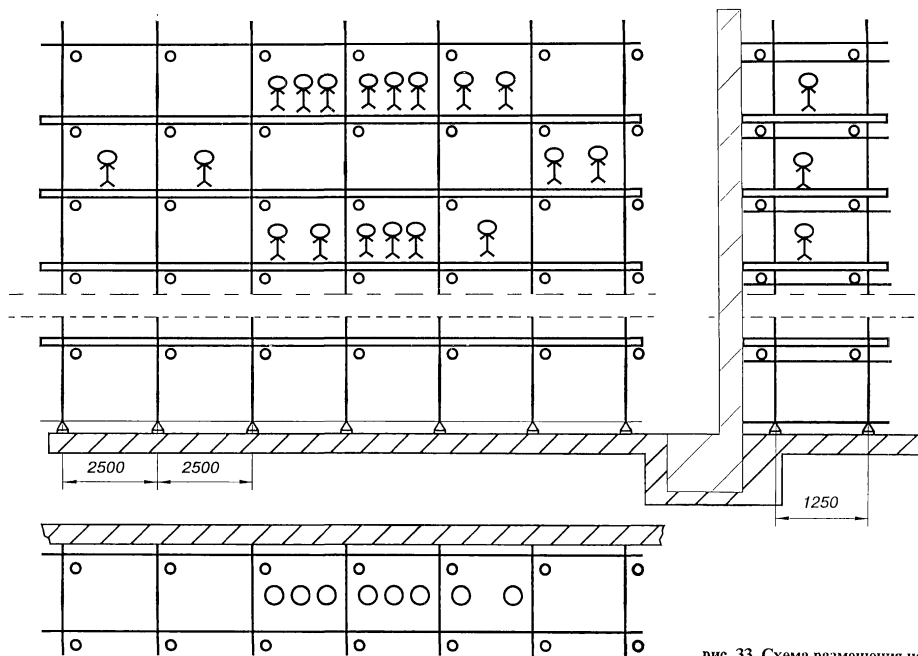
рис. 33. Схема размещения нагрузок.
