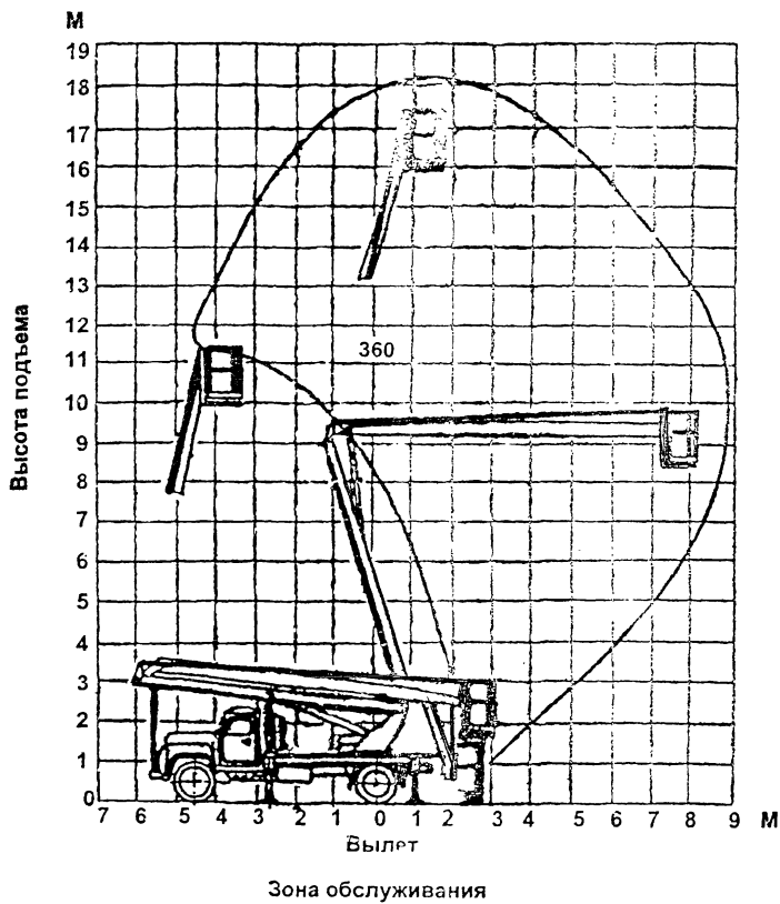
рис. 13. Автогидроподъемник Р-184Н.
