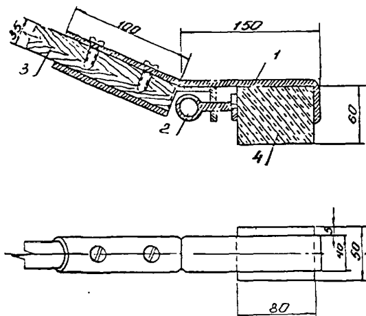
Рисунок 1 – Обойма для крепления лещадь или пемзы
