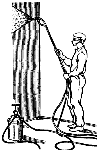
Рисунок 2 – Огрунтовка поверхности стены малярной удочкой
