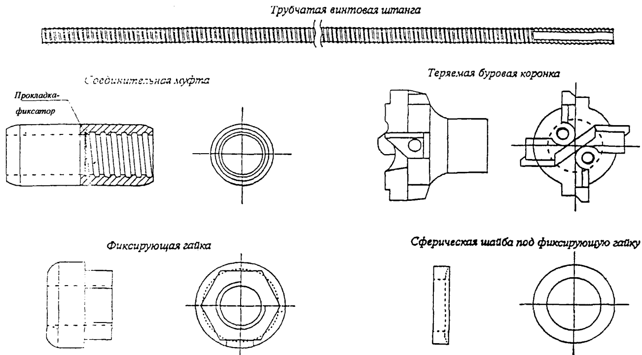
Рисунок 2—Схемы составляющих конструктивных элементов
