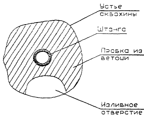
Рисунок 5—Схема устройства пробки в устье скважины
