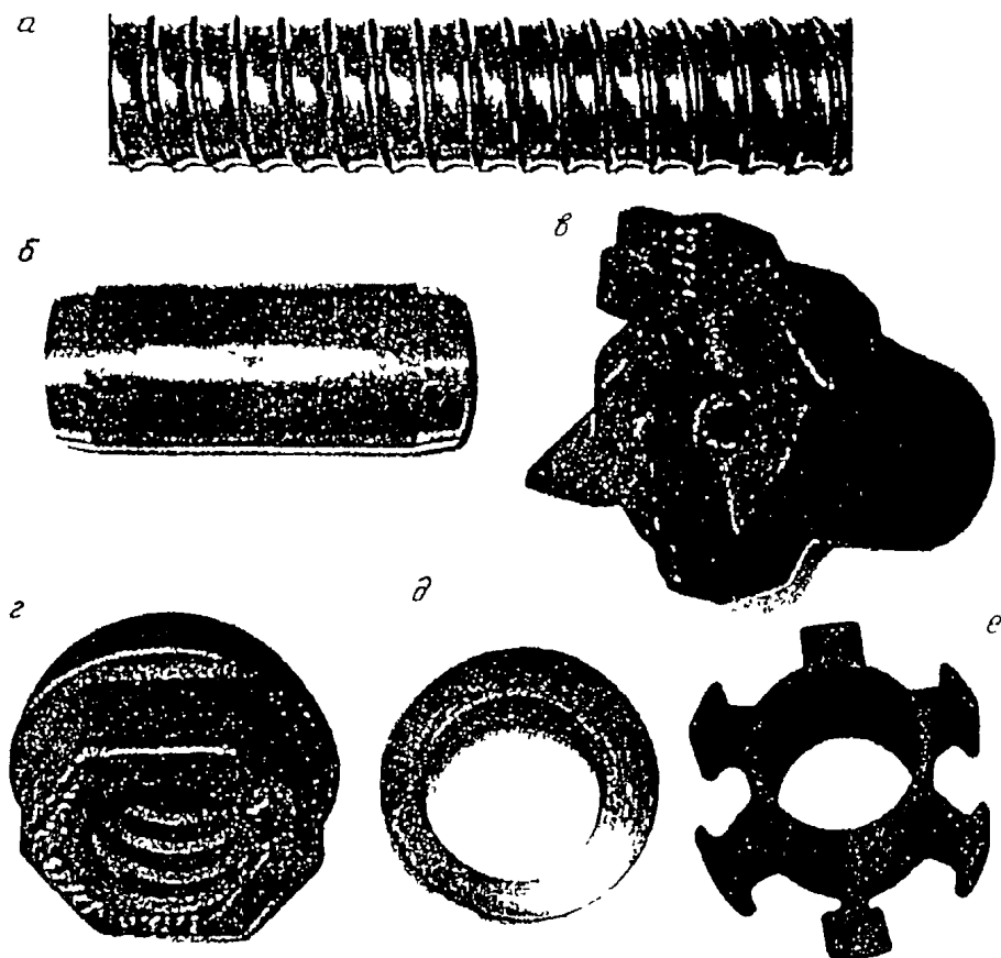
а – полая трубчатая штанга, б – соединительная муфта, в – буровая коронка для глинистых грунтов, г – фиксирующая шайба, д – сферическая шайба, е – центратор
