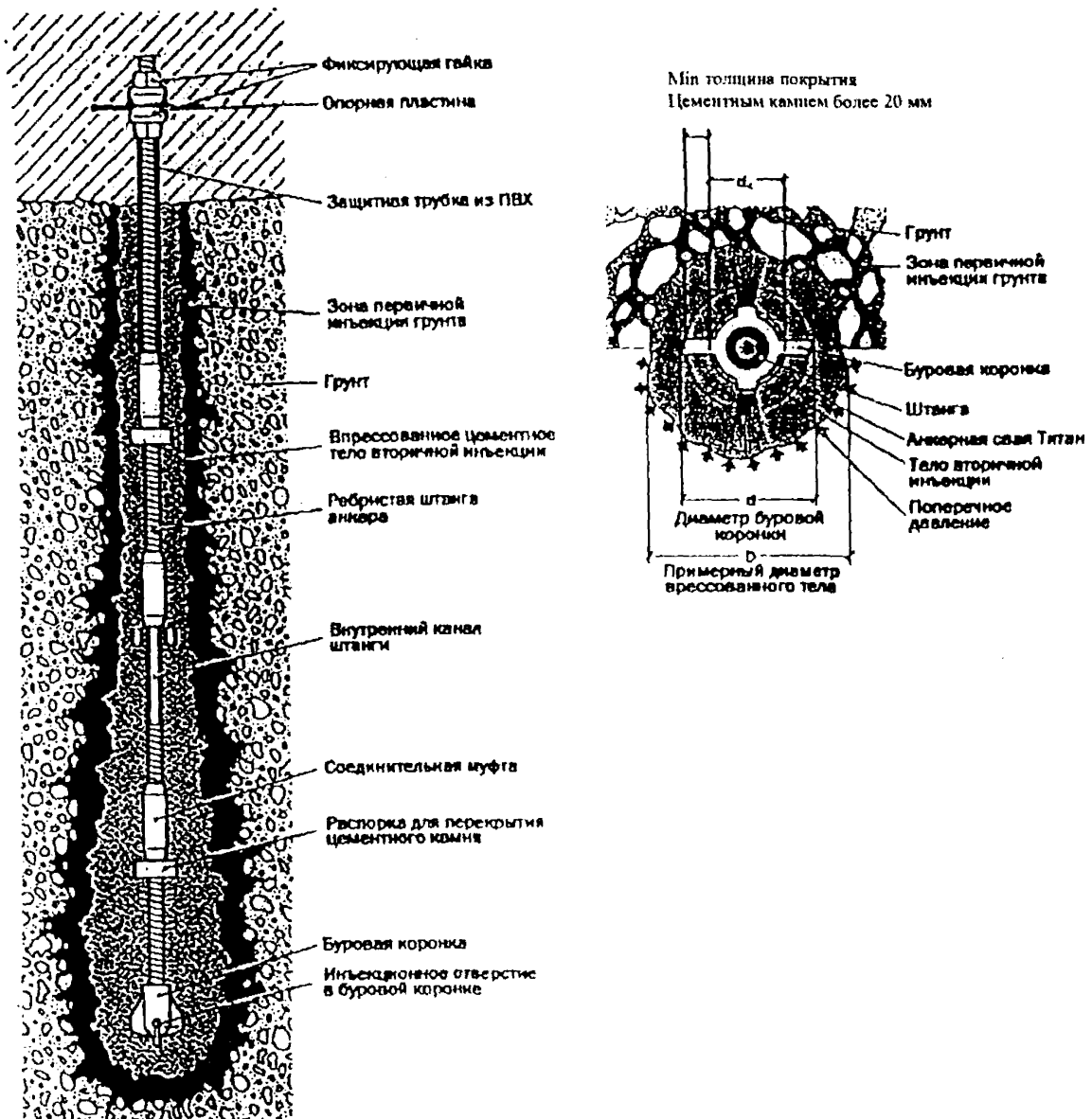
Рисунок 1 — Конструкция анкера (свай) из трубчатых штанг в грунте
