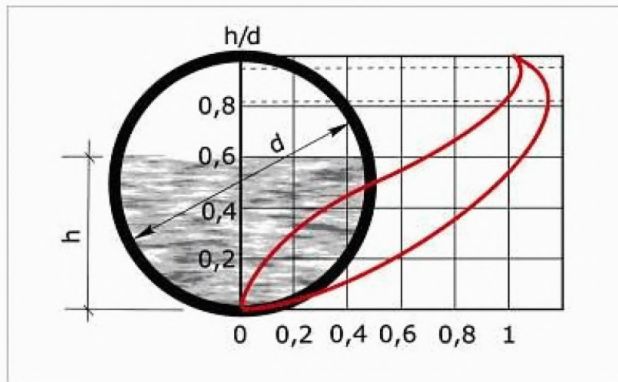
Зависимость расхода q и скорости V от степени наполнения трубопровода h/d .
