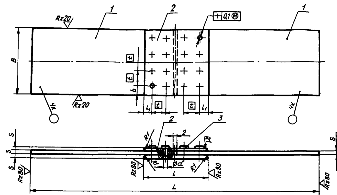
1 - пластина; 2 - накладка; 3 - заклепка Черт. 5
