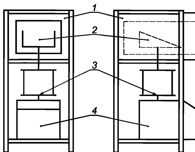
1 — печь; 2 — контейнер для взвешивания внутри печи; 3 — платформа для взвешивания вне печи, соединенная с весами (комнатная температура); 4 — весы
