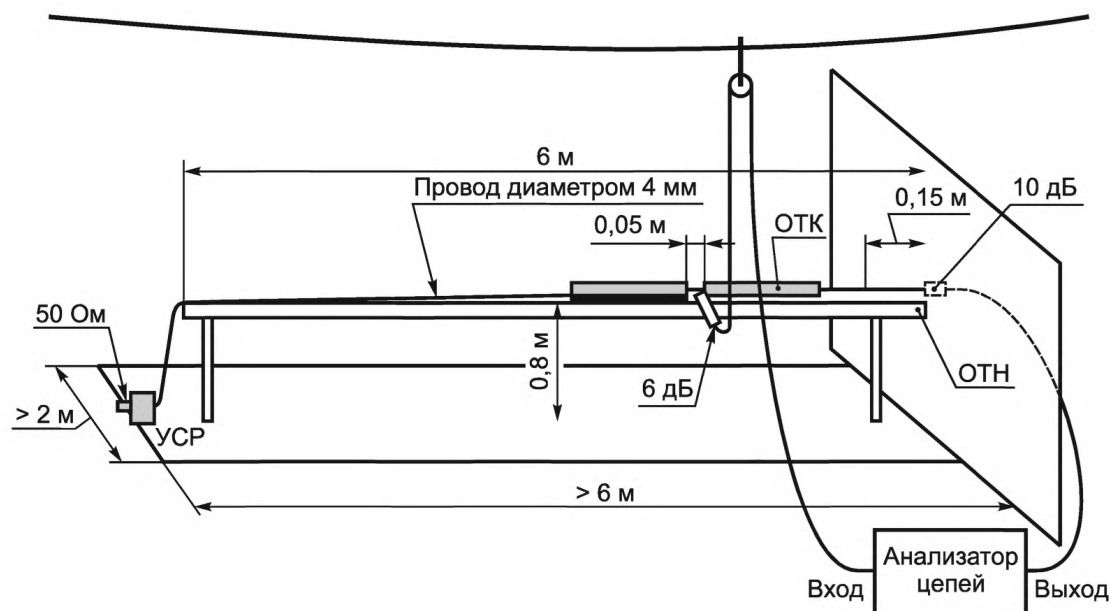
Рисунок Б.1 — Измерительная площадка для калибровки поглощающих клещей основным методом
