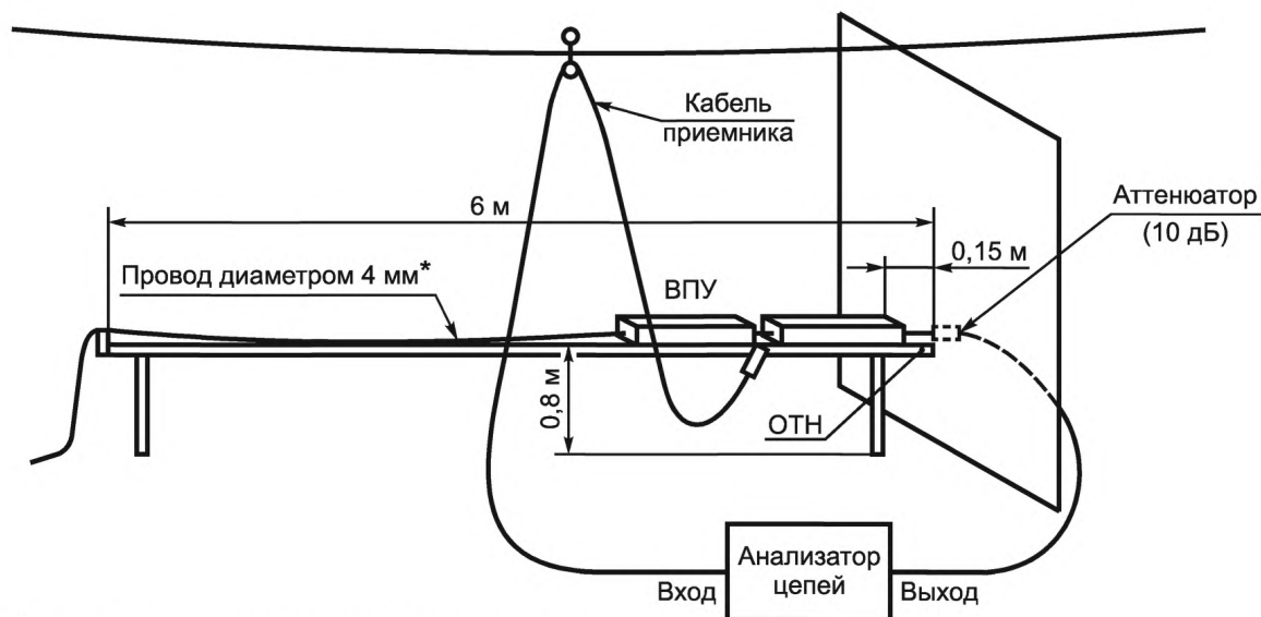
б) Установка для измерений мощности на выходе поглощающих клещей
