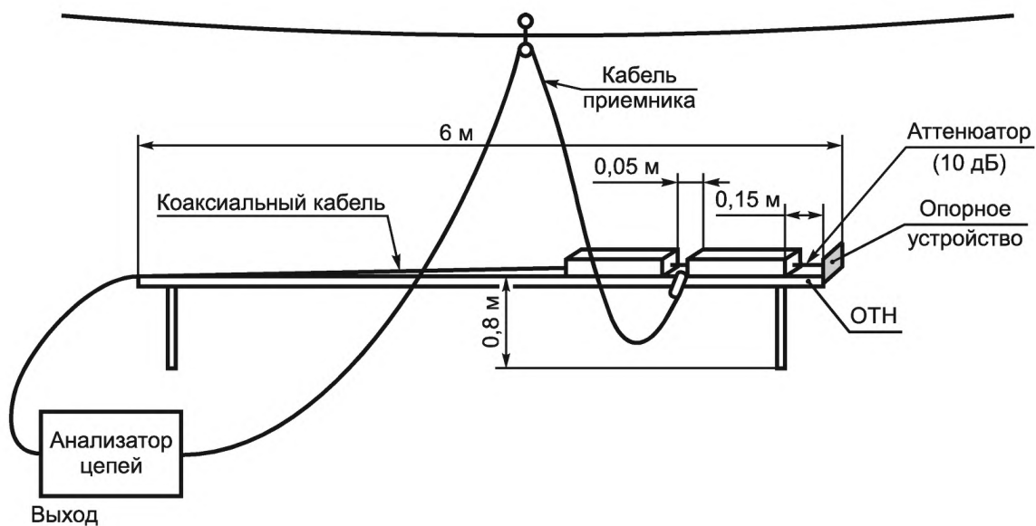
Рисунок Б.6 — Испытательная установка для калибровки поглощающих клещей с помощью опорного устройства
