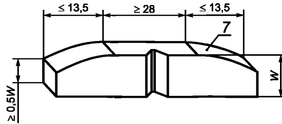
с — Размеры альтернативных образцов
