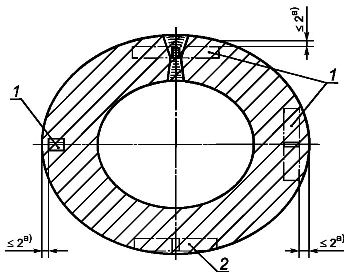
а — Расположение испытательных образцов
