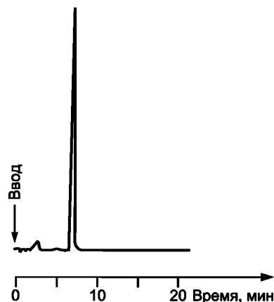
Рисунок 4 — Пример хроматограммы ДНФГ-производного формальдегида
