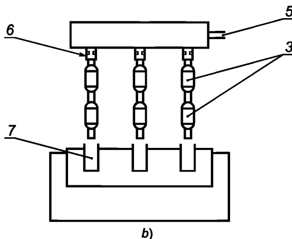
а — устройство для нанесения ДНФГ; б — устройство для сушки картриджей;
