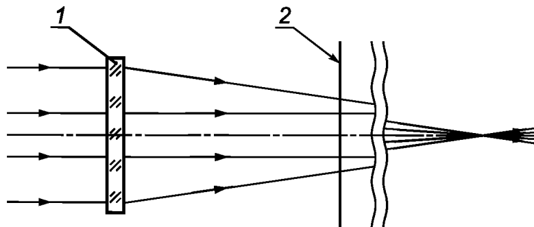
1 — испытуемое очковое стекло; 2 — плоскость измерений
