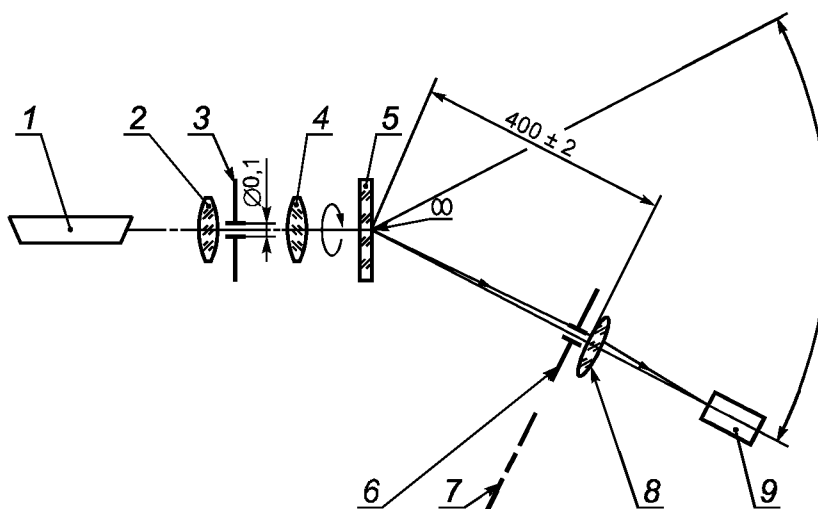
1 — гелий-неоновый лазер; 2, 4, 8 — линзы; 3, 6 — диафрагмы; 5 — исследуемое очковое стекло; 7 — кольцевая диафрагма; 9 — фотоприемник
