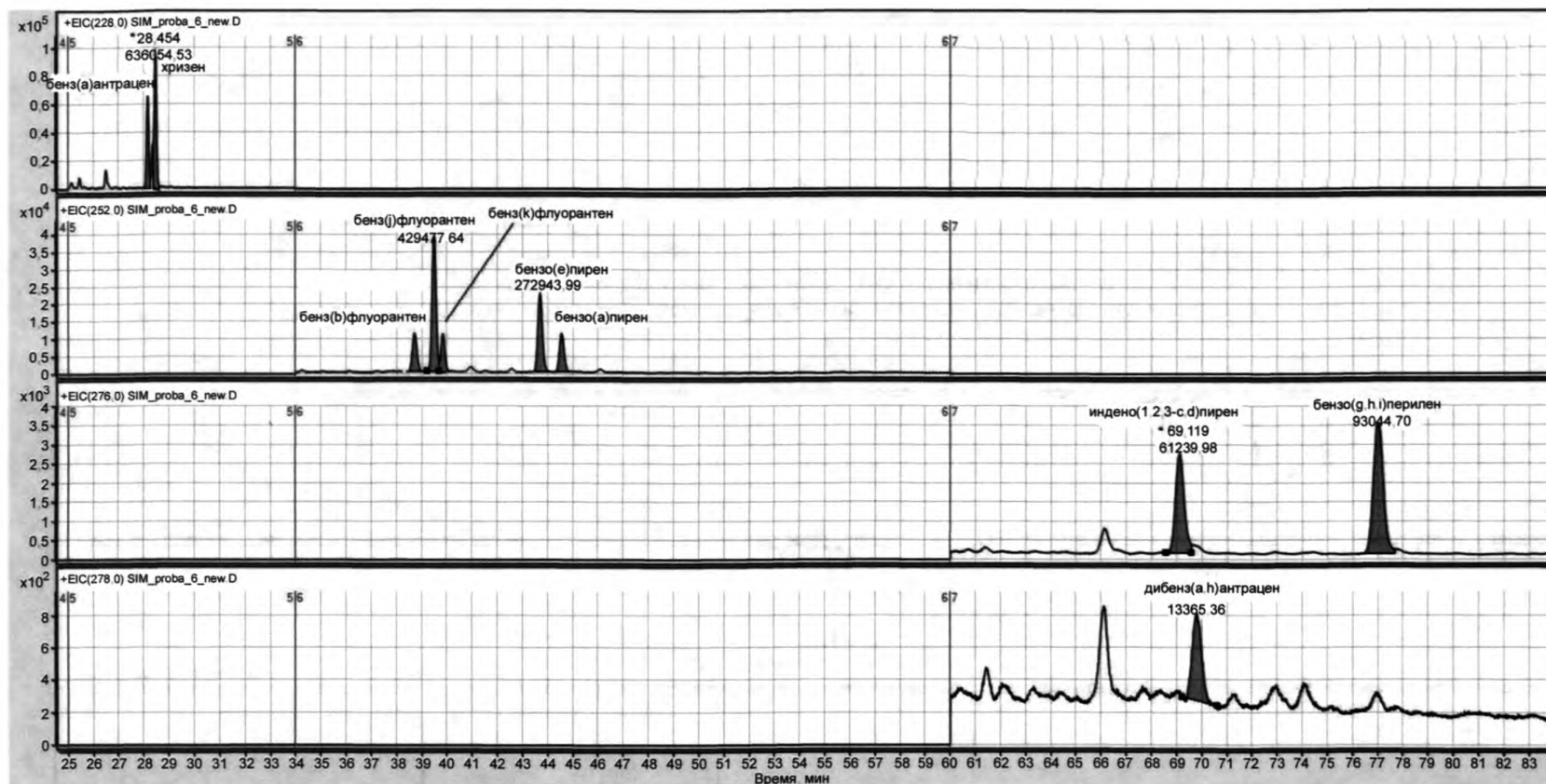
Рисунок Г.2 — Пример хроматограмм стандартного раствора ПАУ в режиме селективного ионного детектирования для бенз(а)антрацена, хризена, бенз(б)флуорантена, бенз(ј)флуорантена, бенз(к)флуорантена, бензо(е)пирена, бензо(а)пирена, индено(1,2,3-с,д)пирена, бензо(г,х,і)перилена и дибенз(а,х)антрацена».
