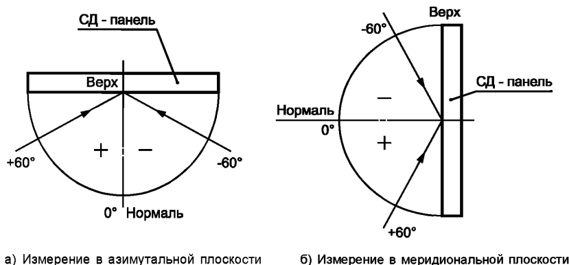
а) Измерение в азимутальной плоскости б) Измерение в меридиональной плоскости Рисунок 9 — Обозначение положительных и отрицательных углов наблюдения для записи в протоколе измерений
