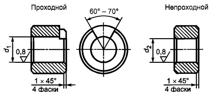
Рисунок А.1 — Проходные и непроходные калибры-кольца для контроля охватываемых концов фитингов
