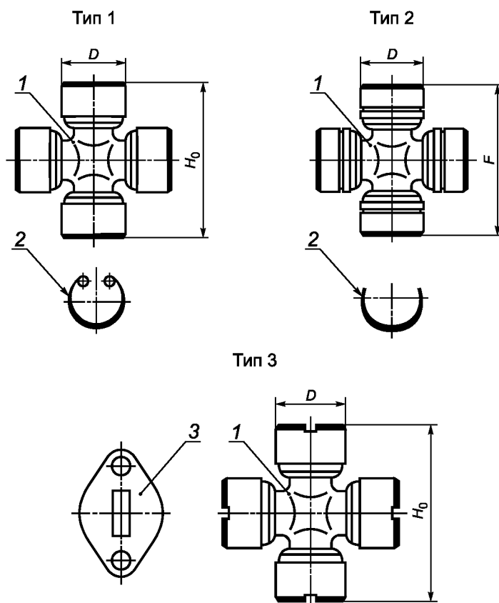
1 — крестовина; 2 — стопорное кольцо; 3 — пластина
