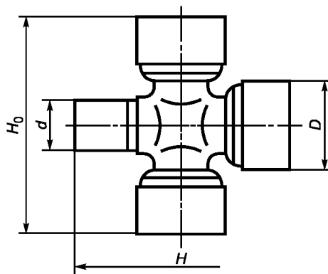
Рисунок 1 — Крестовина карданного шарнира
