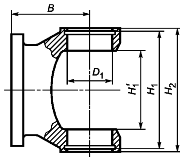
Рисунок 3 — Вилка карданного шарнира
