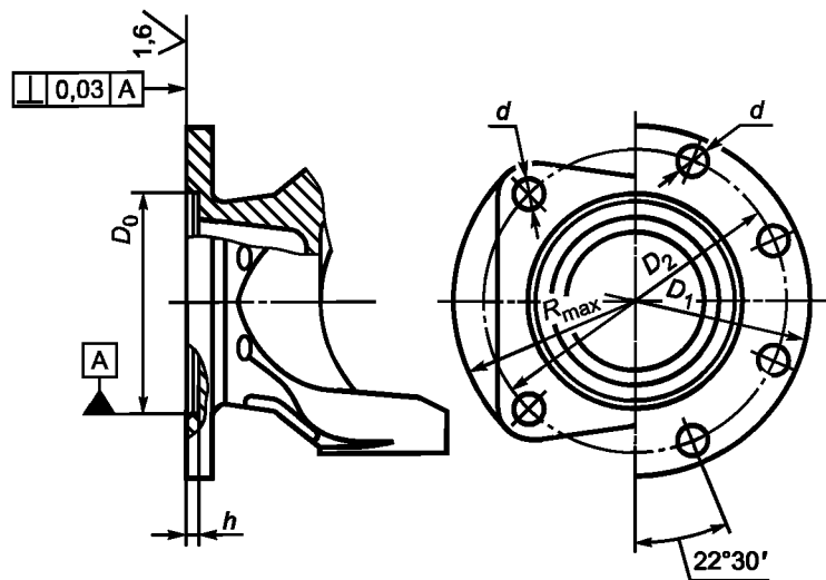
Рисунок 5 — Типы фланцев-вилок карданных шарниров с присоединительными поверхностями
