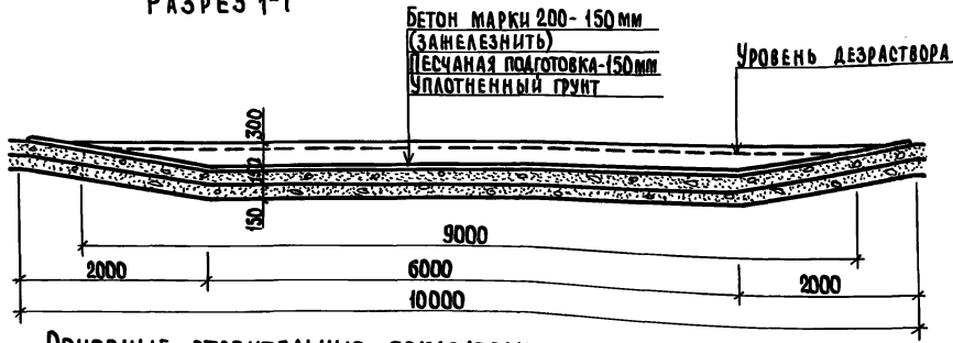
РАЗРЕЗ 1-1
