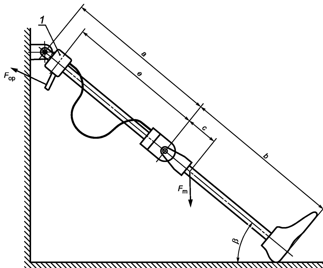
Рисунок D.4 — Образец вида с по D.3.1 (коленные узлы с замком протезных устройств) при испытании по D.6.4
