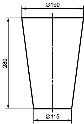
Рисунок С.3 — Размеры образца трансфеморальной приемной гильзы
