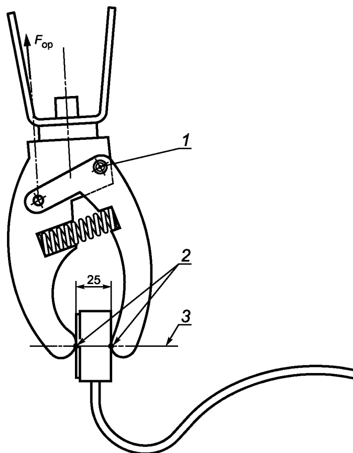
1 — шарнир; 2 — центроиды зон контакта; 3 — ось измерения датчика силы; F_{op} — управляющая сила, действующая параллельно оси переходника (если иное не установлено изготовителем)
