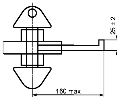
Рисунок А.7 — Длина рукоятки
