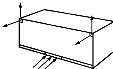
Рисунок 11 — Подъем за боковые угловые фитинги (способ 3)
