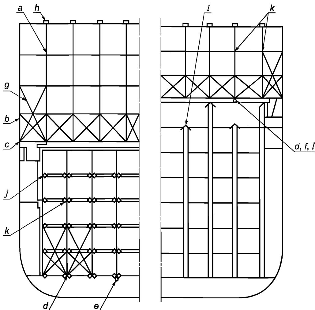
Рисунок 22 — Пример типового оборудования для крепления контейнеров
