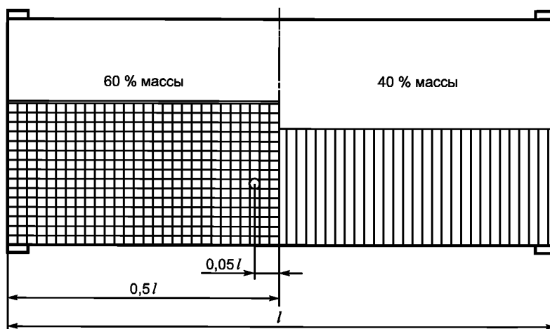
Рисунок 1 — Распределение нагрузки
