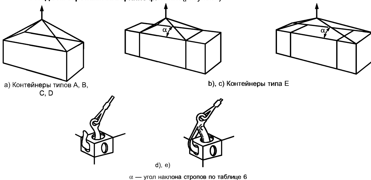
Рисунок 4 — Подъем стропами за верхние фитинги контейнера
