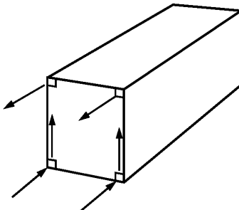
Рисунок 12 — Подъем за торцевые угловые фитинги (способ 1)
