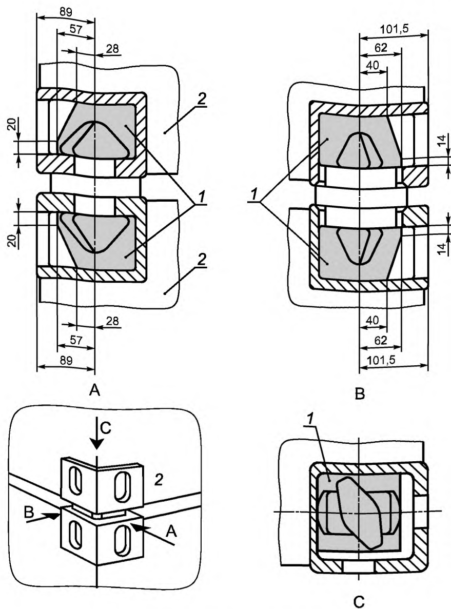
Рисунок D.7 — Ограниченная часть полости углового фитинга
