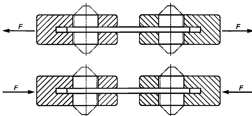
Рисунок С.9 — Испытание на растяжение и сжатие
