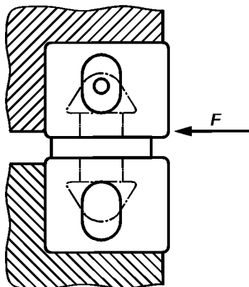
Рисунок А.13 — Испытание стопора на срез
