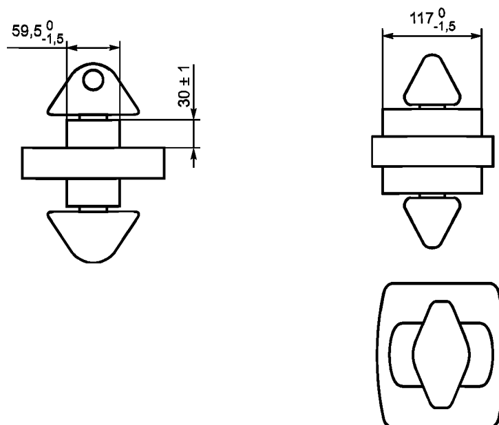
Рисунок А.8 — Размеры выступов
