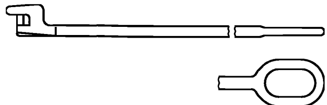
Рисунок D.3 — Контейнерная штанга с оголовком
