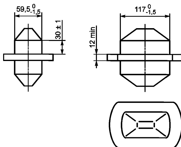
Рисунок С.4 — Размеры штабелирующего конуса
