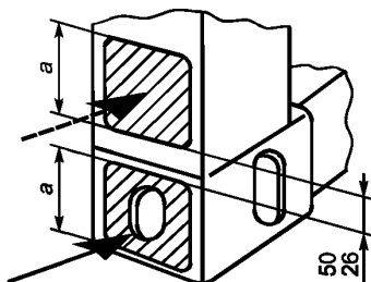
Рисунок 13 — Подъем за торцевые угловые фитинги (способ 2)
