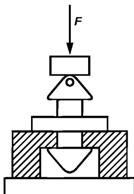
Рисунок А.12 — Испытание конуса стопора на сжатие
