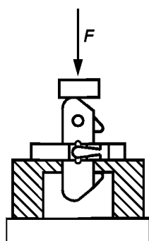
Рисунок В.11 — Испытание конуса стопора на сжатие
