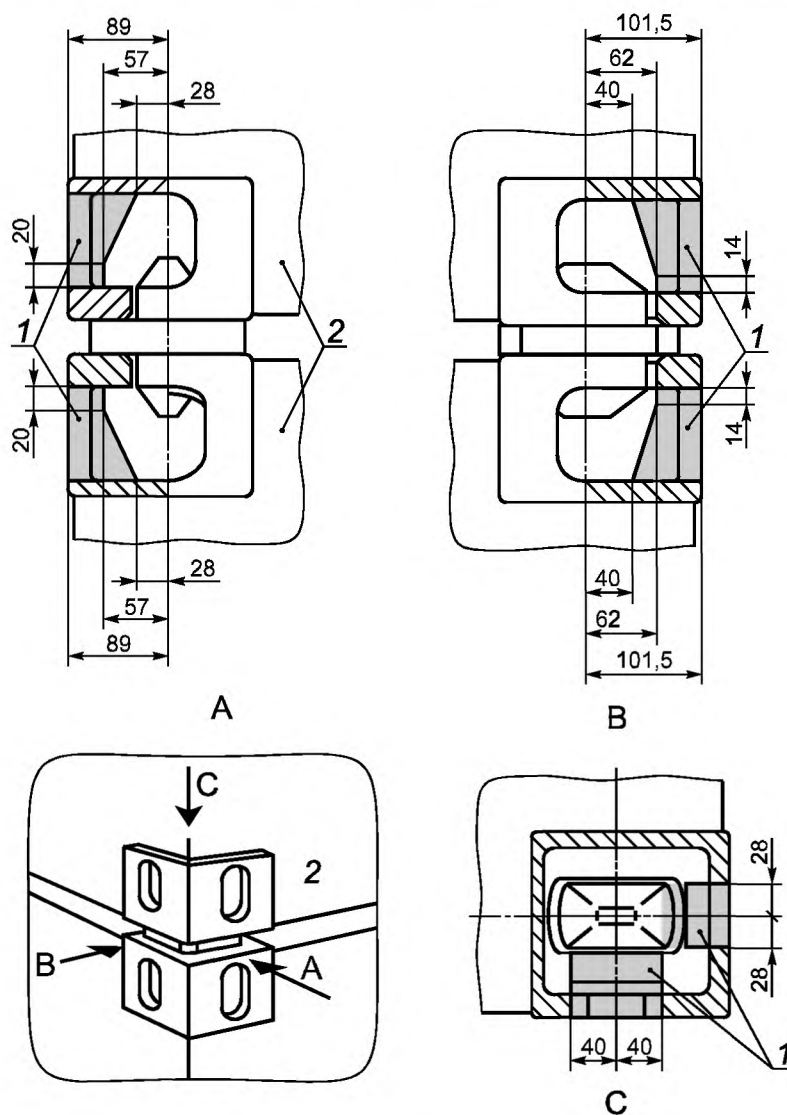
Рисунок С.3 — Ограниченная часть полости углового фитинга
