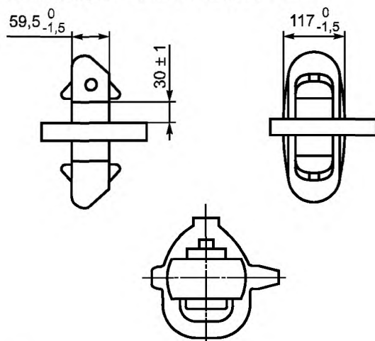
Рисунок В.7 — Размеры выступов
