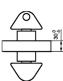
Рисунок А.6 — Промежуточная пластина
