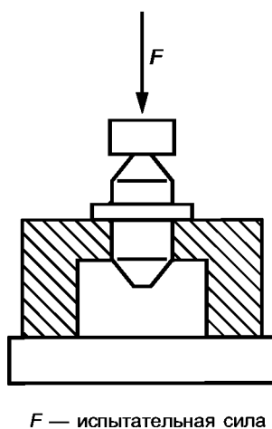
Рисунок С.7 — Испытание конусов на сжатие
