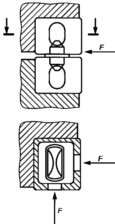
Рисунок С.8 — Испытание конусов на срез
