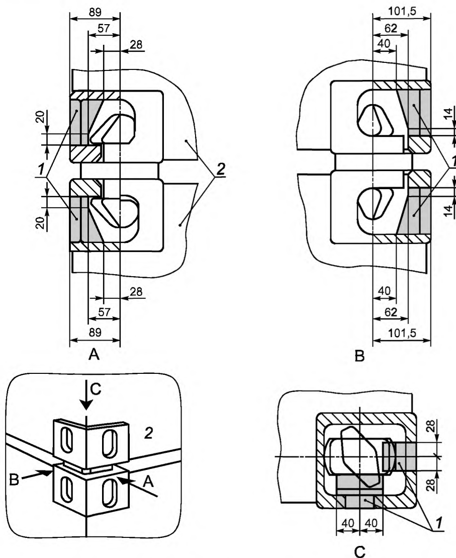
Рисунок A.5 — Ограниченная часть полости углового фитинга
