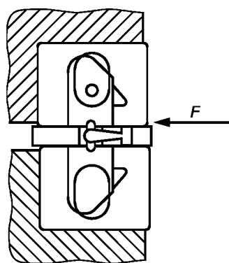
Рисунок В.12 — Испытание стопора на срез
