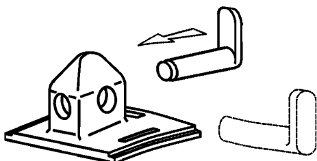
Рисунок 27 — Стопорный конус с закладным пальцем (штырем)
