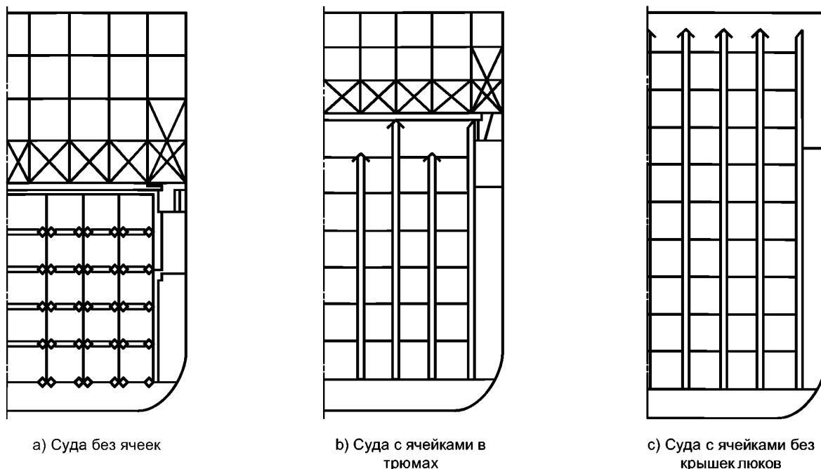
Рисунок 21 — Примеры конструкций судов-контейнеровозов
