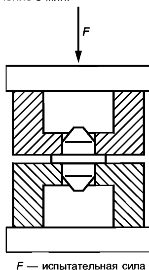
Рисунок С.6 — Испытание промежуточной пластины на сжатие
