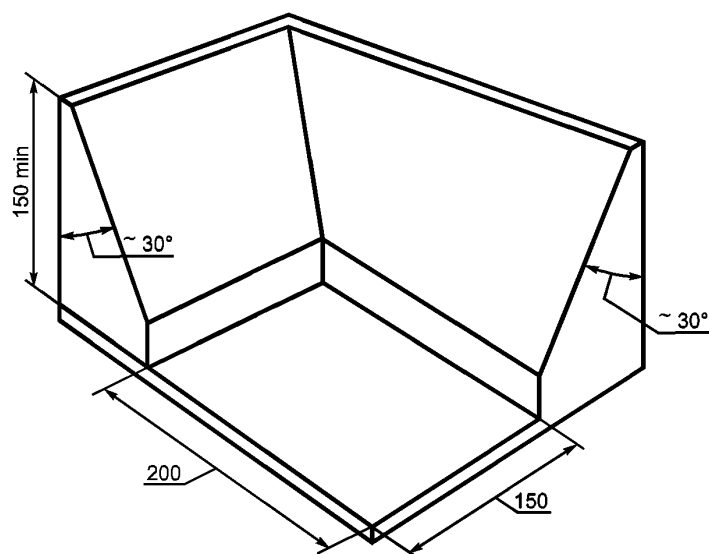
Рисунок 24 — Пример угловой направляющей с горизонтальным упором
