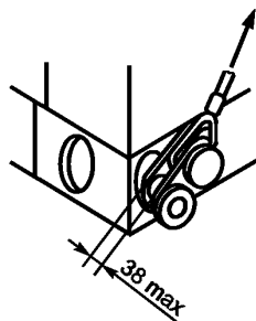
Рисунок 7 — Крепление стропа к нижнему фитингу
