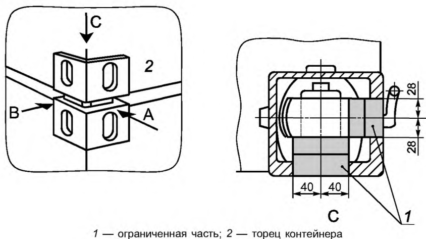
Рисунок В.4, лист 2
