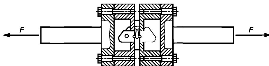
Рисунок В.9 — Испытание стопора на растяжение
