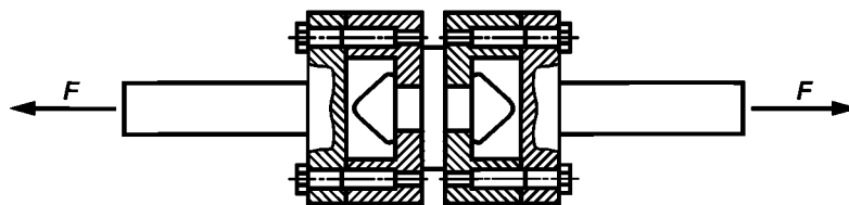
Рисунок A.10 — Испытание стопора (твистлока) на растяжение
