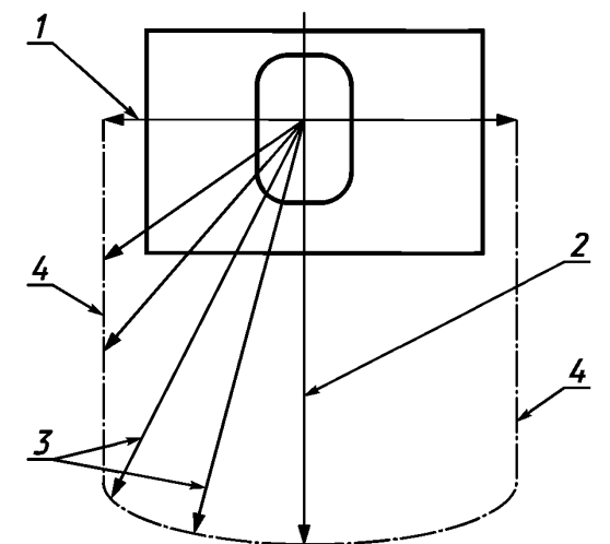
1 — горизонтальная нагрузка 150 кН; 2 — вертикальная нагрузка 300 кН; 3 — предельные (результатирующие) нагрузки; 4 — граница зоны распределения нагрузок
