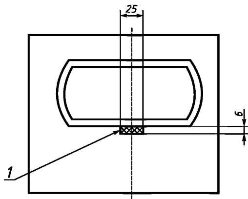
1 — площадка, воспринимающая нагрузку при неправильной установке контейнера
