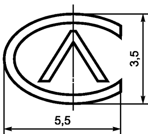
Рисунок 2 — Сталь с пределом пропорциональности \sigma_{\text{e}} \geq 700 \text{ МПа}
