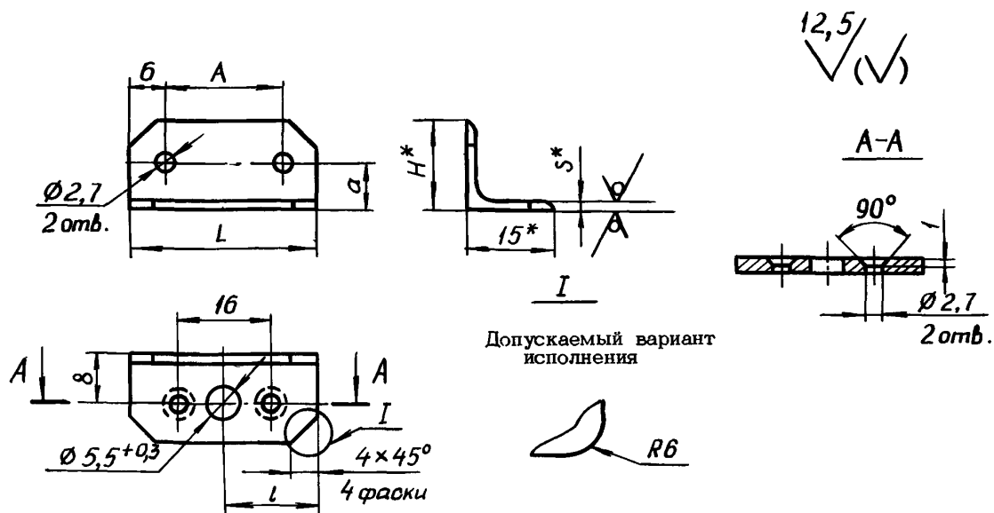
Размеры, мм
