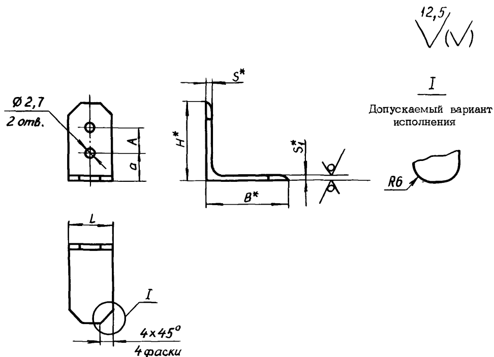
Размеры, мм
