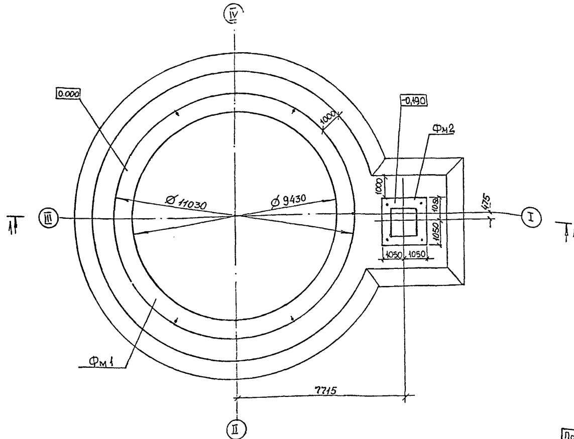
Схема расположения фундаментов.
