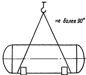
Сосуды объемами от 10 до 25 м³
