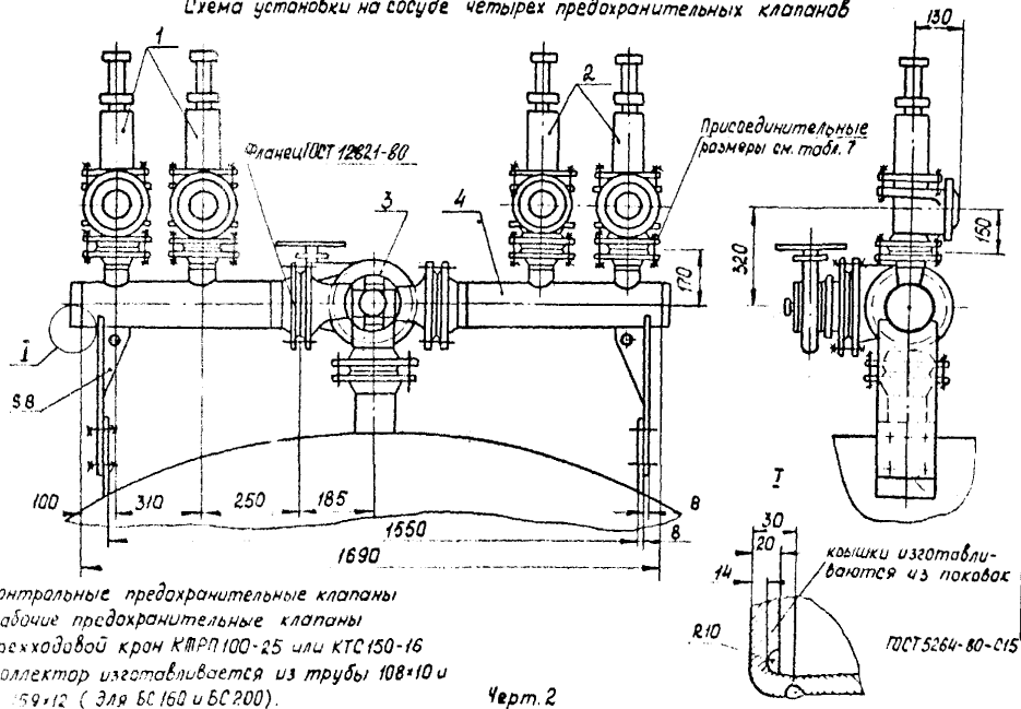
Схема установки на сосуде четырех предохранительных клапанов
