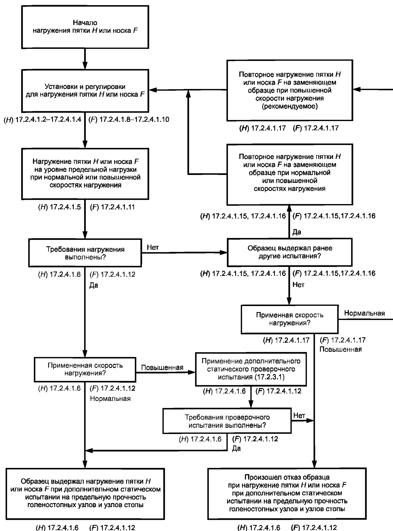
Рисунок 18 — Блок-схема дополнительного статического испытания на предельную прочность голеностопных узлов и узлов стоп, установленного в 17.2.4.1
