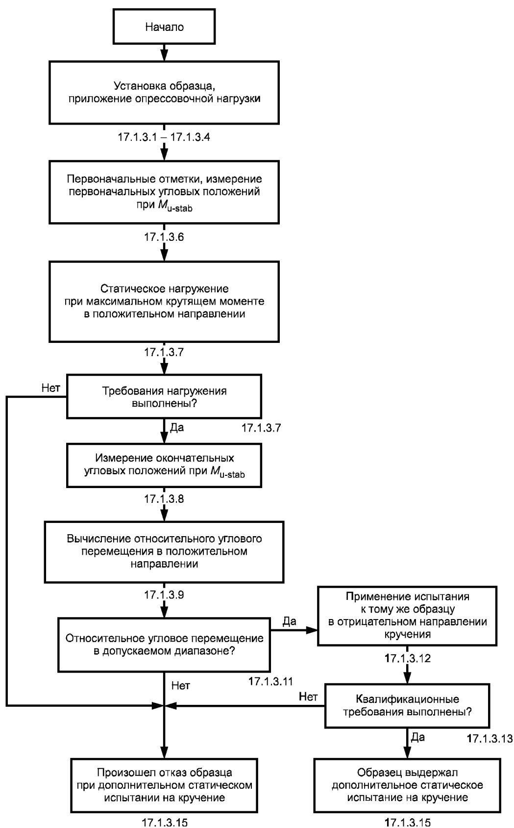
Рисунок 16 — Блок-схема дополнительного статического испытания на кручение, установленного в 17.1.3
