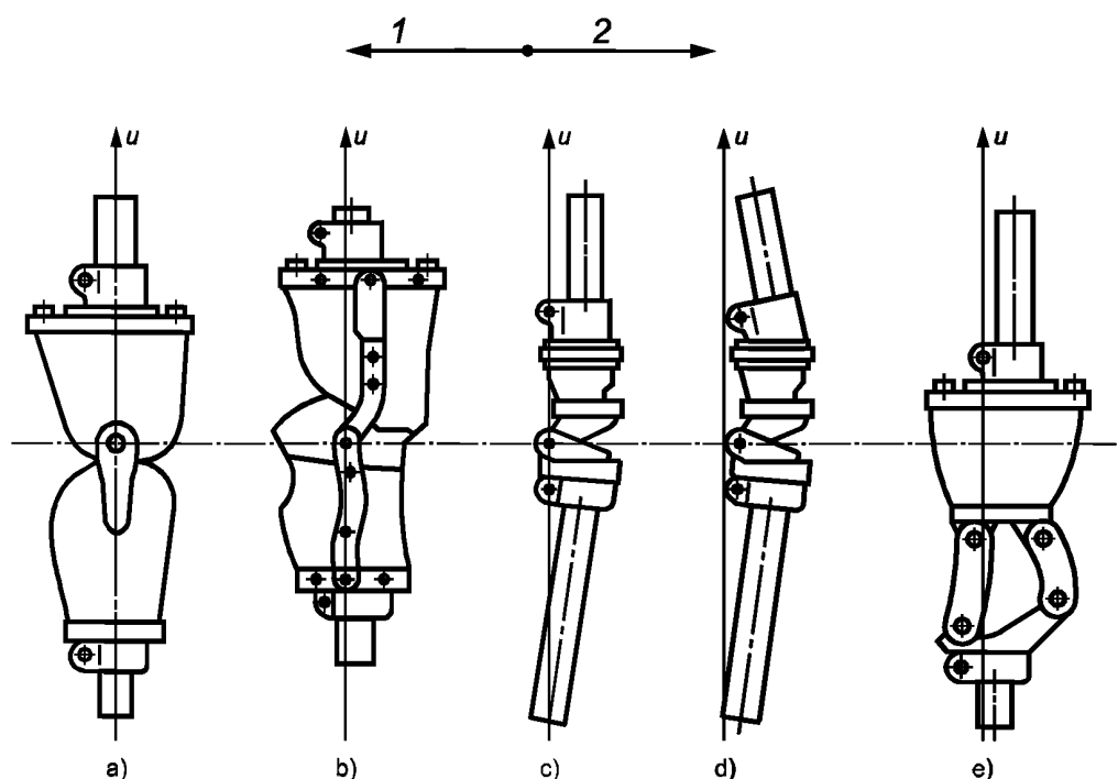
а), б), в) — расположение действительной центральной линии коленного узла, указанного в 6.7.5.1; д), е) — расположение действительной центральной линии коленного узла, указанного в 6.7.5.2; 1 — ориентация 1: постериорное (в направлении тыльной стороны); 2 — ориентация 2: anteriорное (в направлении лицевой стороны)
