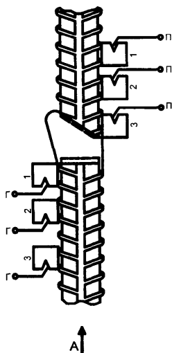
Рис. 6. Проведения контроля сварных соединений теньевым методом.
