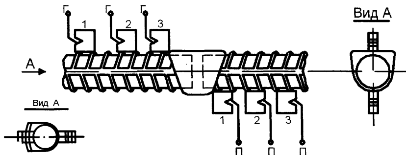
Рис. 6. Проведения контроля сварных соединений теньевым методом.
