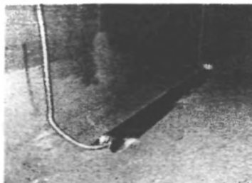
Установка сенсора с термопарой на опоре моста
