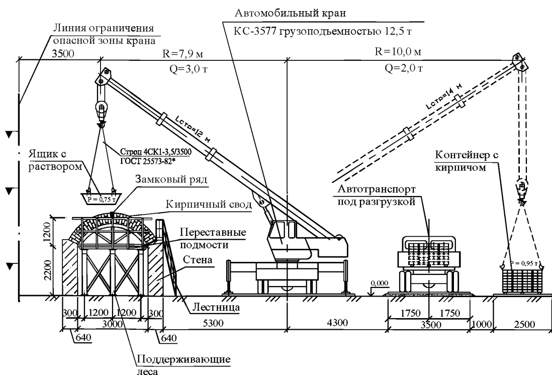
Рисунок 5 – Схема разгрузки автотранспорта и подачи материалов в рабочую зону
