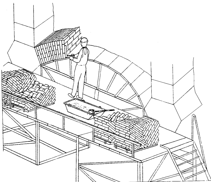
Рисунок 9 – Выверка кладки
