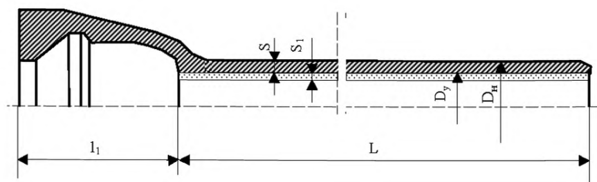
Рисунок А.1 – Труба раструбная под соединение «Универсал»
