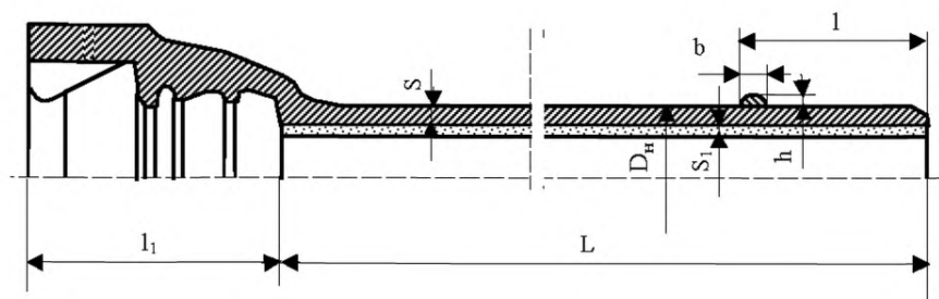
Рисунок А.2 – Труба раструбная под соединение «ВРС»
