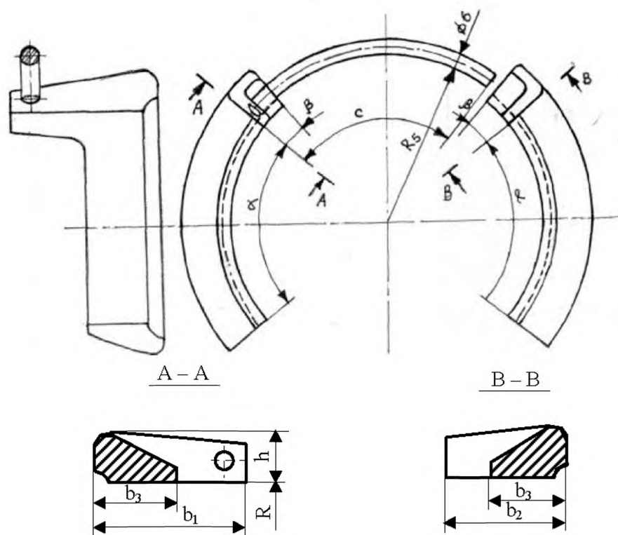
Рисунок А.8 – Стопор из высокопрочного чугуна (под соединение «ВРС»)
