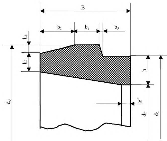
Рисунок А.4 – Уплотнительное резиновое кольцо (под соединение «Универсал»)
