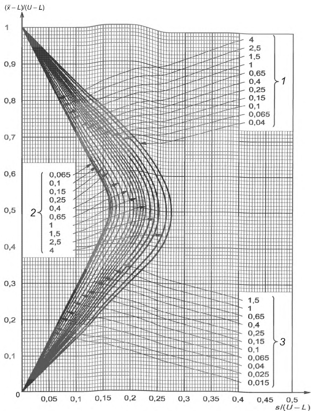
Рисунок 28 — График s-M. Приемочные кривые для объединенного контроля с двумя пределами поля допуска и общим AQL. «s» метод. Код объема выборки М (объем выборки 95) (для ослабленного контроля код объема выборки Р)
