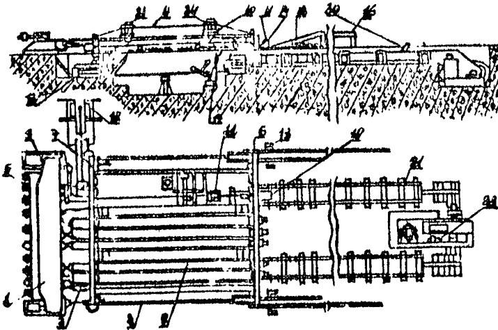
Рис.2. Схема формовочной машины для изготовления многоспанельных панелей при конвейерном способе производства:
