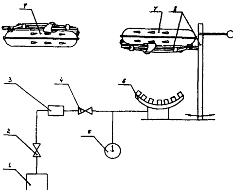
Рисунок 2. Схема огневой установки по определению устойчивости противогАЗа к воздействию пламени:
