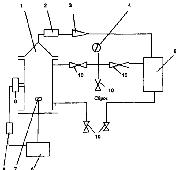
Установка для определения максимального давления при воспламенении БПИ:
