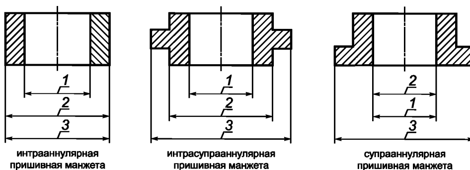
Рисунок 2 — Типы пришивных манжет
