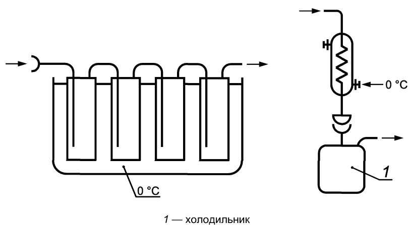
Рисунок В.5 — Схемы двух охлаждающих систем
