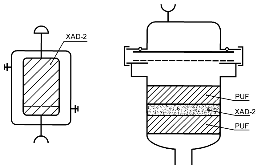
Рисунок В.6 — Схемы двух картриджей с сорбентом
