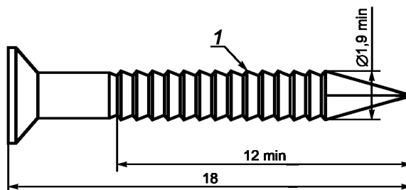
Рисунок 1 — Стандартный каблучный гвоздь
