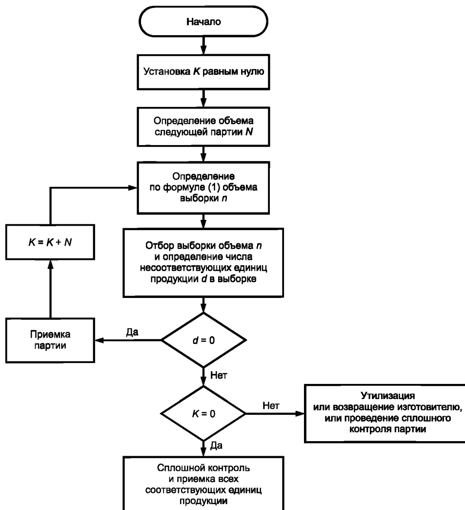
Рисунок 1 — Блок-схема стандартной процедуры приемки
