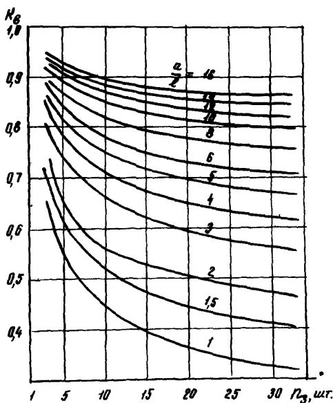
Рис.9. Зависимость коэффициента экранирования горизонтальных заземлителей K_g от числа электродов n_3 при различных отношениях \frac{a}{\ell} : a - расстояние между заземлителями, м; \ell - длина заземлителей 3 м, глубина установки 1,5 м
