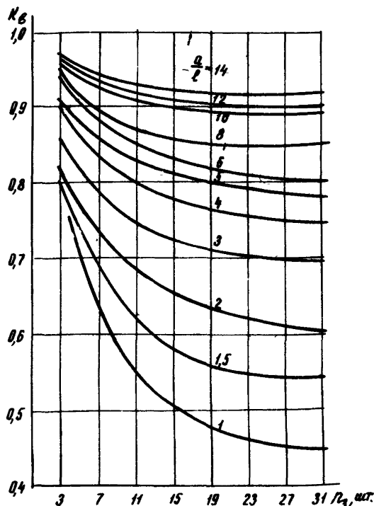
Рис.8. Зависимость коэффициента экранирования горизонтальных заземлителей в коксовом активаторе K_B от числа электродов n_3 при различных отношениях \frac{a}{l} . a - расстояние между заземлителями, м; l - длина заземлителей 1,4 м, глубина установки 1,7 м
