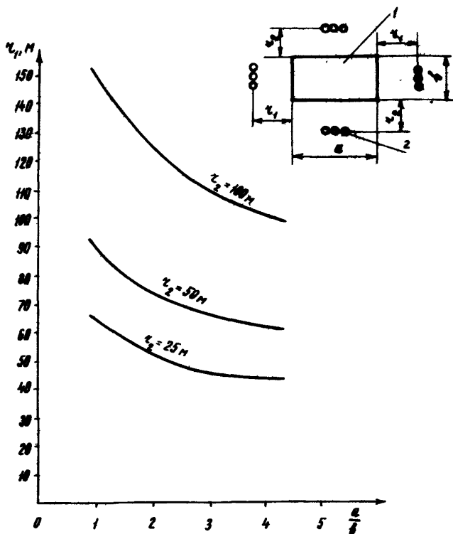
Рис.5. Зависимость величины отнoса сосредоточенных анодных заземлений от соотношения сторон площадки:
