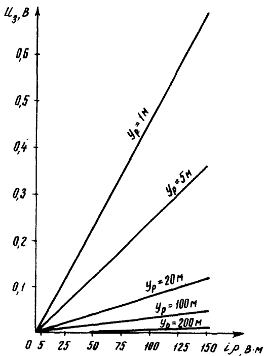
Рис.3. Зависимость потенциала земли U_3 от напряженности поля E_r сооружения длиной 20 м в точке, удаленной от сооружения на расстоянии y_P
