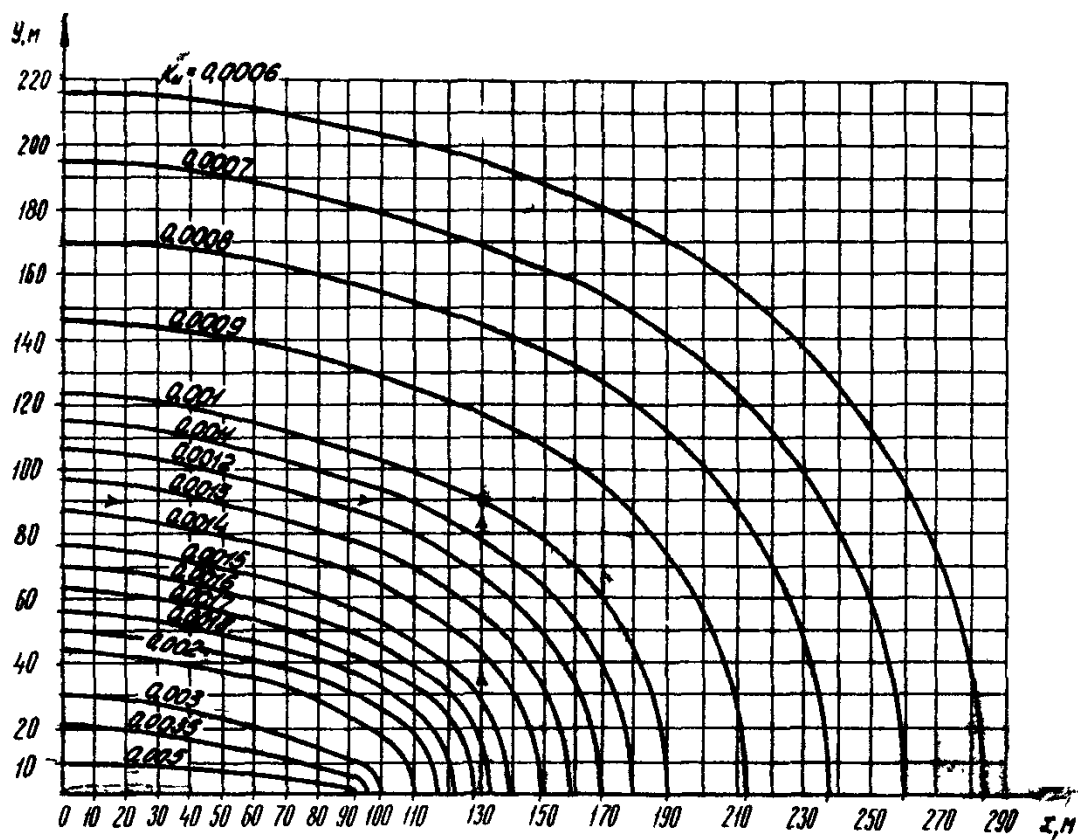
Рис.26. Коммуникация длиной 180 м
