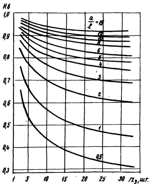
Рис.7. Зависимость коэффициента экранирования вертикальных заземлителей K_\phi от числа электродов n_3 при различных отношениях \frac{a}{\ell} :
